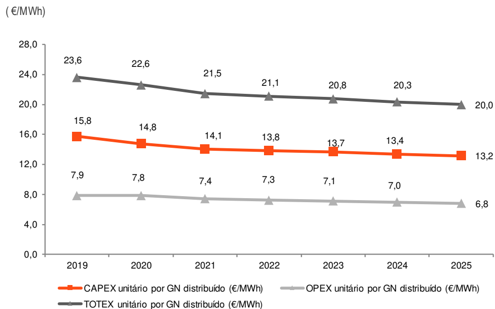
Figura 34 - Evolução do custo unitário €/MWh
