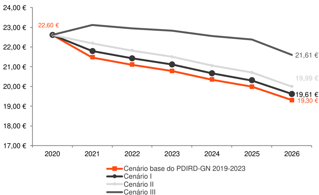
Figura 36- Evolução do TOTEX por MWh 2021-2025
