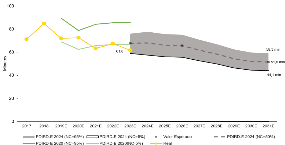
Figura 5-4 - Evolução do Indicador SAIDI MT entre 2017 e 2023, e previsão até 2031
