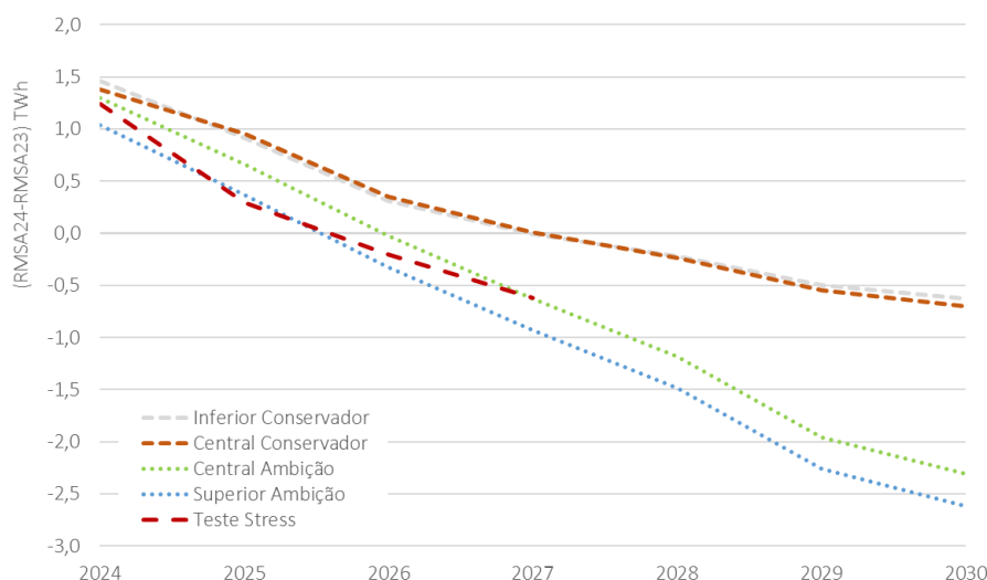
Figura 3-2 – Diferença da evolução dos cenários de consumo entre o RMSA-E 2024 e RMSA-E 2023
