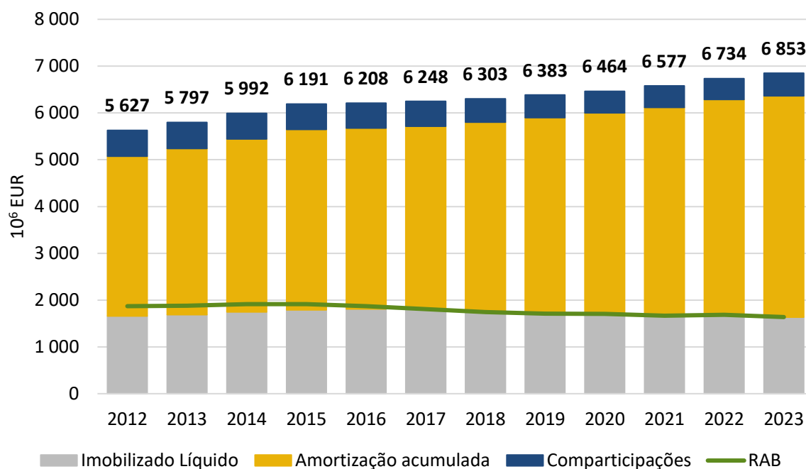
Figura 6-4 - Evolução do ativo em AT/MT
