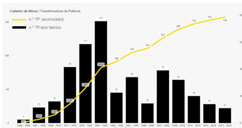
Figura 5-2 - Ano de fabrico dos transformadores de potência da RND
