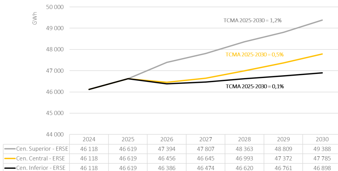
Figura 3-3 – Cenários da ERSE para a veiculação de energia elétrica na RND em AT e MT, de 2024 a 2030
