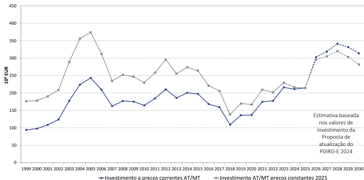
Figura 6-3 - Evolução do investimento na rede de AT/MT 25
