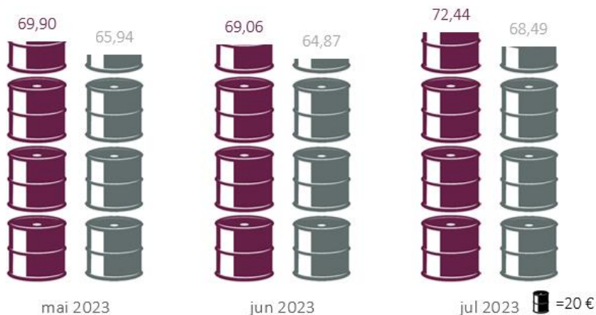
Figura 1-2 – Preços médios mensais de BFO e WTI, FOB
