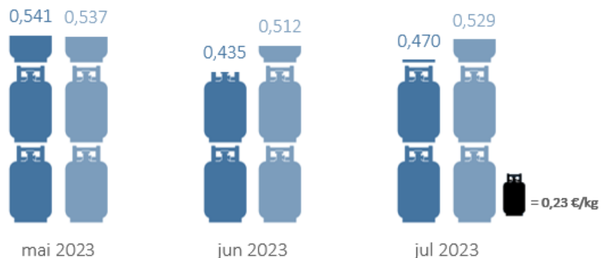
Figura 2-4 – Preços médios mensais de propano e butano
