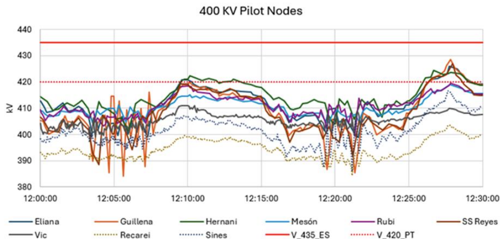
Figura 6 - Evolução da tensão das 12:00 às 12:30 CEST nas principais subestações de transporte de 400 kV em Espanha e Portugal. [fonte: Telemedidas a cada 4" da Red Eléctrica e REN]
