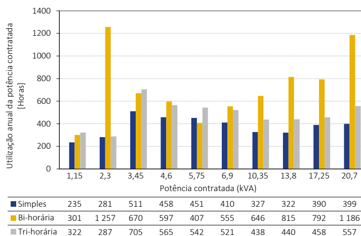
Figura 10-12 - Utilização da potência contratada, por opção tarifária e por escalão de potência ( \leq 20,7 kVA)*
