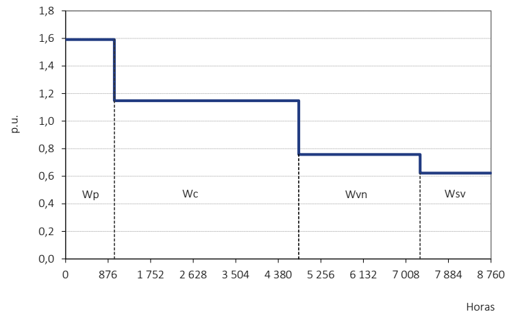
Figura 9-9 - Diagrama de carga dos clientes em BTN (&gt; 20,7 kVA), discriminado por período tarifário
