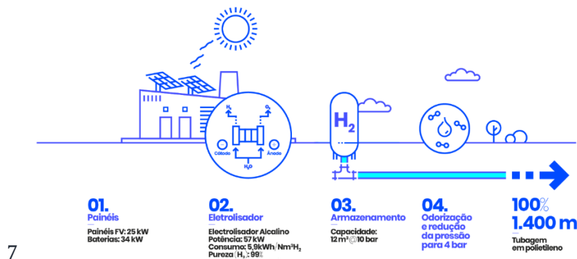
Figura 31 - Esquema de produção de hidrogénio e veiculação na tubagem de PE - Esquema interno
