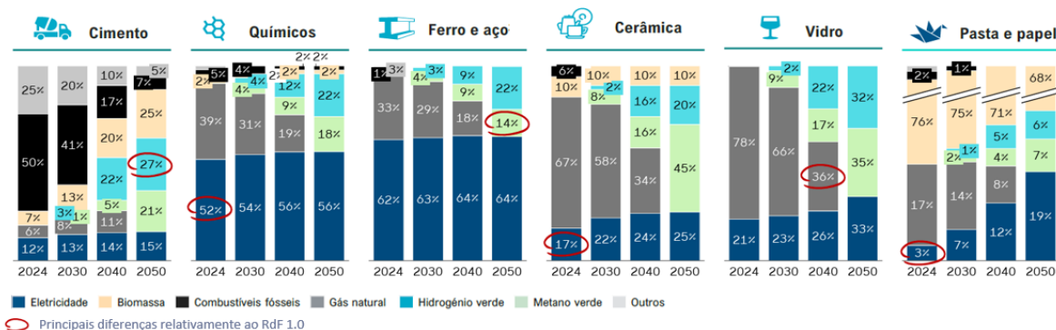
Figura 30 - Potencial evolução do mix energético das principais indústrias nacionais – RdF 2.0
