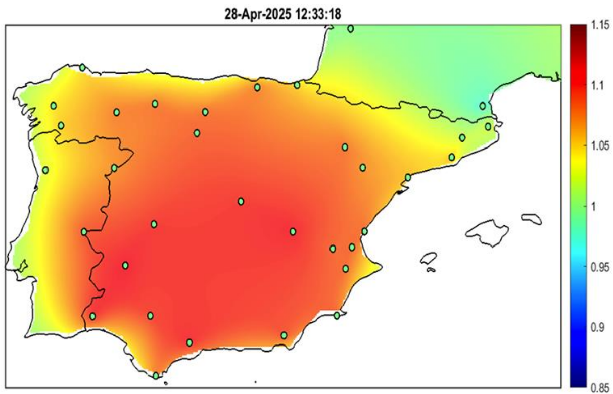
Figures 12a, 12b & 12c – Mapas térmicos da tensão na rede de transporte a 400 kV em valores por unidade (p.u.) em cada segundo depois do disparo dos três conjuntos de geradores (fonte: dados PMU da Red Eléctrica, REN e RTE)
