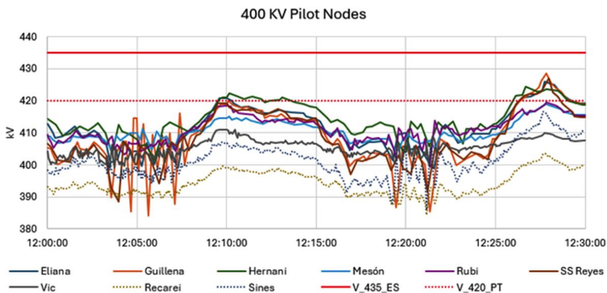
Figura 10a - Evolução da tensão das 12:00 às 12:30 CEST nas principais subestações de transmissão de 400 kV em Espanha e Portugal. [fonte: Telemidas a cada 4" da Red Eléctrica e REN]
