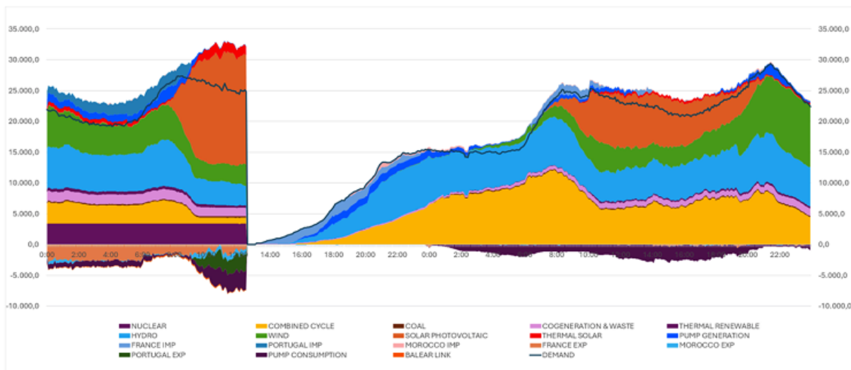
Figura 16a – Mix de geração e consumo em Espanha nos dias 28 e 29 de abril
