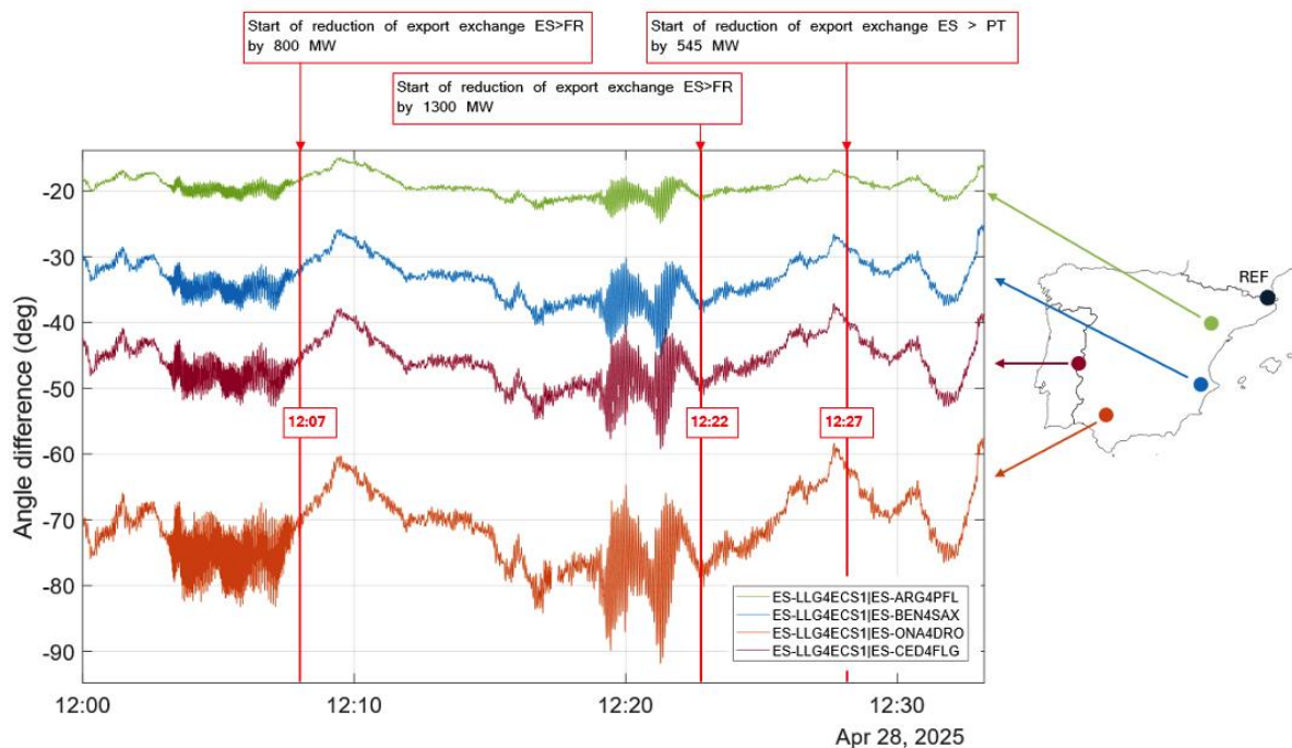
Figura 9 – Evolução da diferença do ângulo de tensão após as 12:00 CEST, e o efeito das contramedidas, em 4 locais da Península Ibérica (fonte: dados da PMU da Red Eléctrica)
