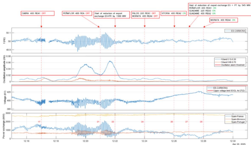
Figura 7 – Dados característicos das segundas oscilações e aumento de tensão (fonte: Taxa de amostragem WAMS de 100 ms na subestação de Carmona de 400 kV) e contramedidas
