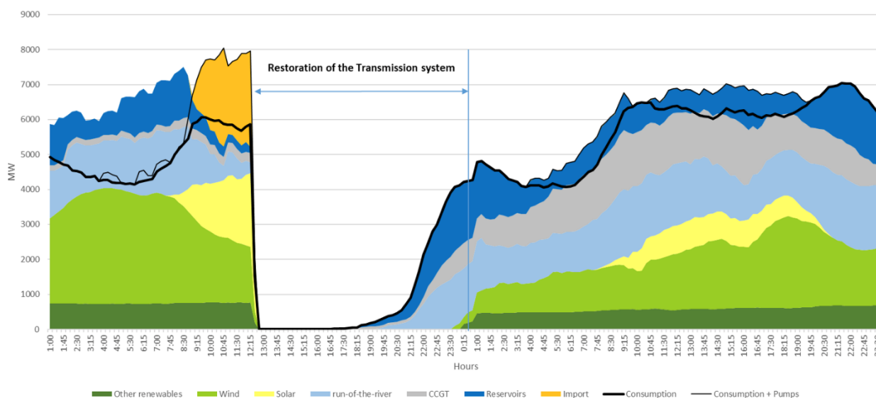
Figura 16b – Mix de geração e consumo em Portugal nos dias 28 e 29 de abril
