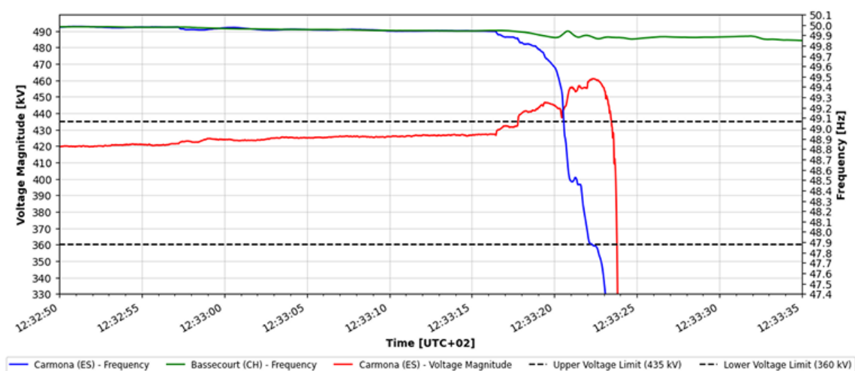
Figure 14 – Evolução da frequência e tensão na subestação de Carmona (Espanha) e da frequência no resto da Europa continental (subestação de Bassencourt, Suíça) durante o incidente (fontes : Red Eléctrica, Swissgrid)
