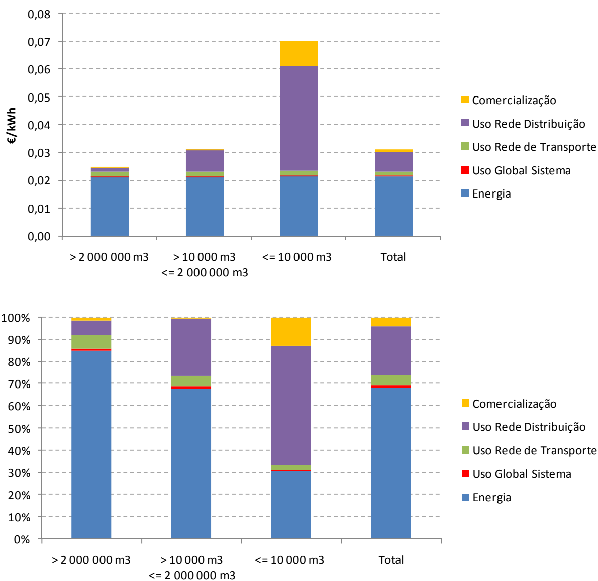
Figura 6-1 – Decomposição dos preços das tarifas de Venda a Clientes Finais pelas várias actividades da cadeia de valor do sector do gás natural
