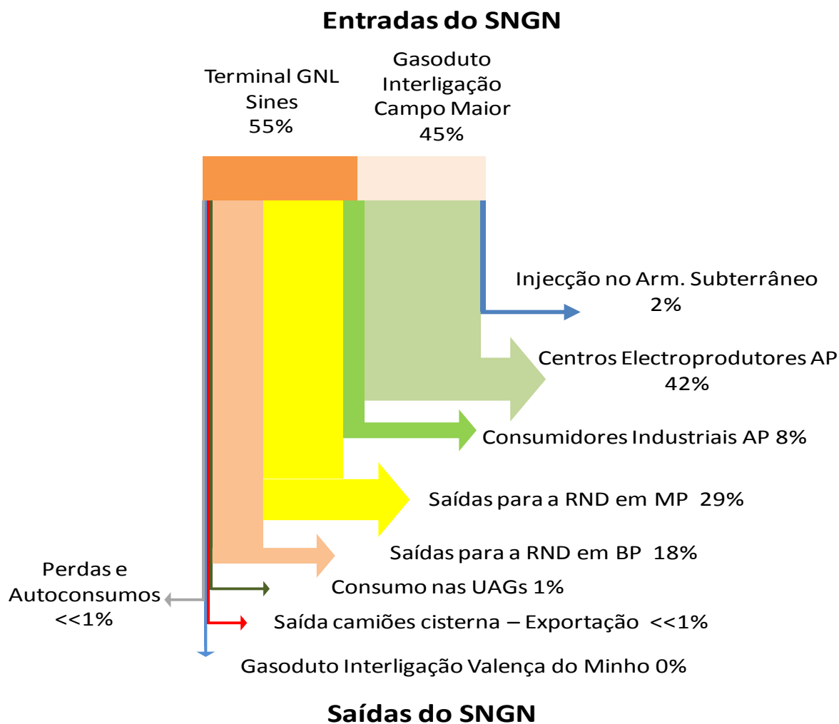
Figura 8-1 – Fluxos de energia do sector do gás natural
