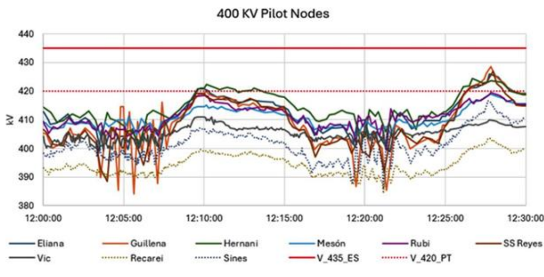
Figura 6 - Evolução da tensão das 12:00 às 12:30 CEST nas principais subestações de transmissão de 400 kV em Espanha e Portugal. [fonte: Telemididas a cada 4" da Red Eléctrica e REN]
