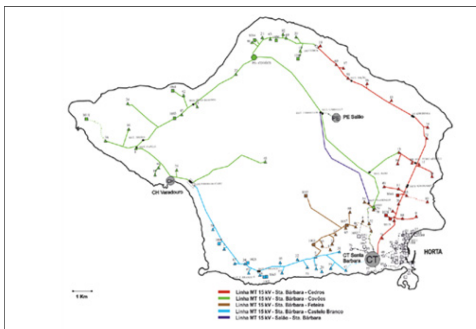
Figura 2-17 – Mapa das redes elétricas da ilha do Faial a 31/12/2023
