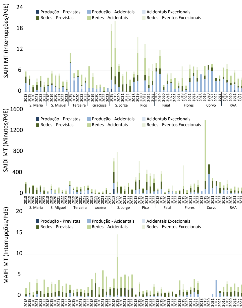
Figura 2-65 – Evolução dos principais indicadores gerais de continuidade da rede MT na RAA
