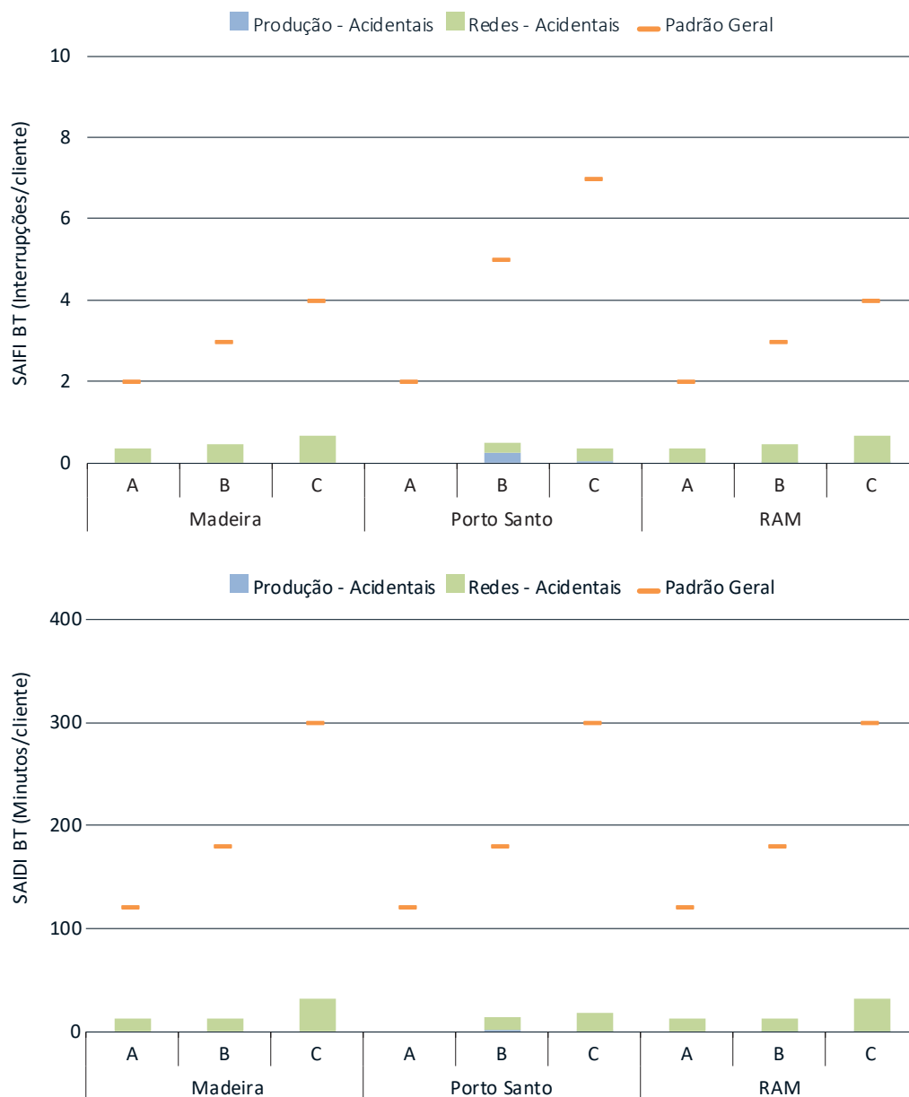
Figura 2-72 – SAIFI BT e SAIDI BT na RAM – comparação com o padrão, em 2023
