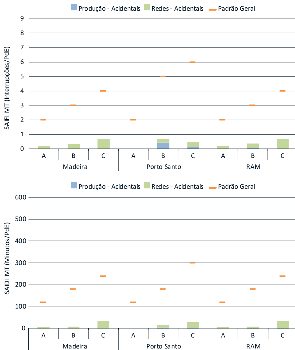
Figura 2-71 – SAIFI MT e SAIDI MT na RAM – comparação com o padrão, em 2023
