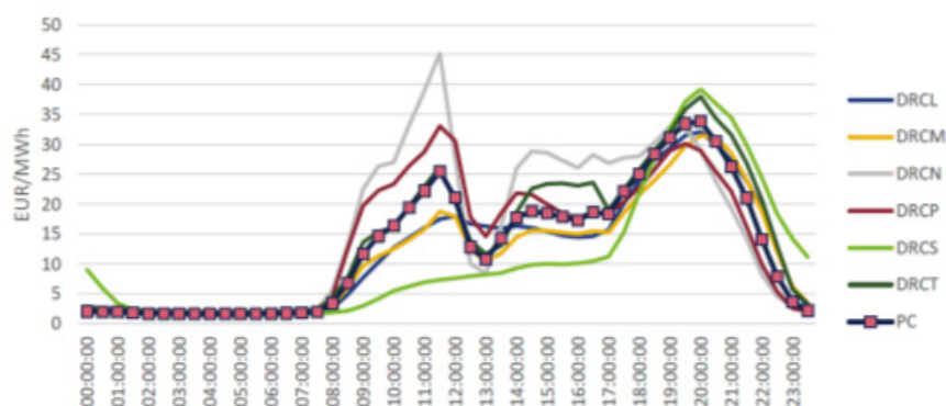
Figura 5-6 – Diagrama horário dos custos das redes, por área de rede 240
