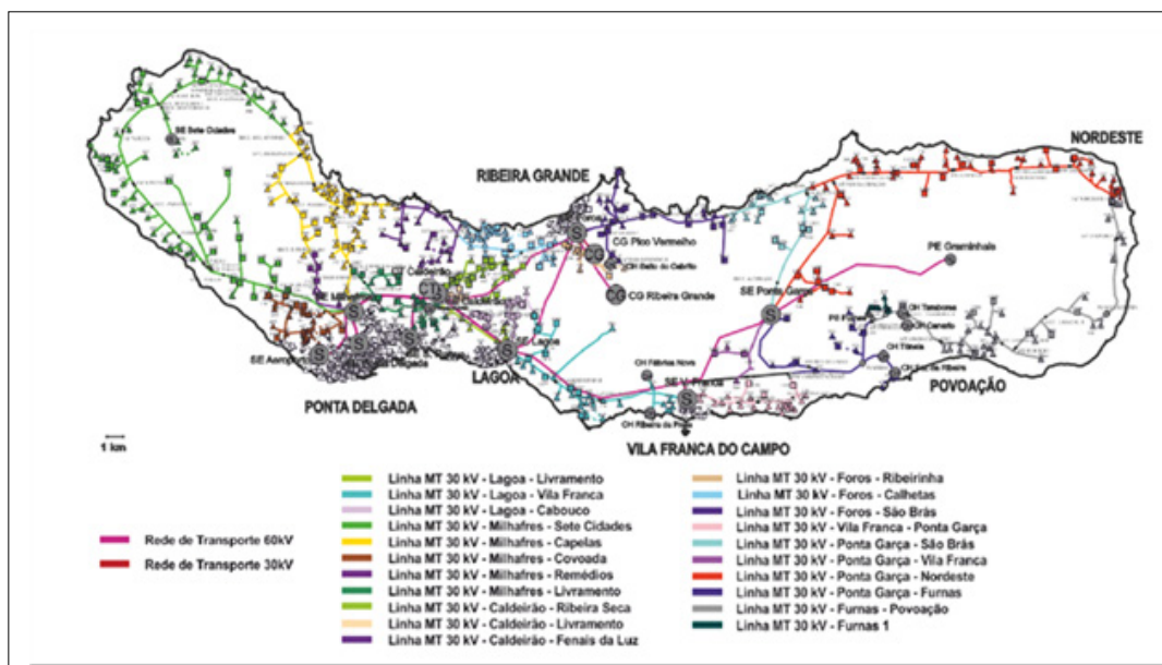
Figura 2-12 – Mapa das redes elétricas da ilha de São Miguel a 31/12/2023
