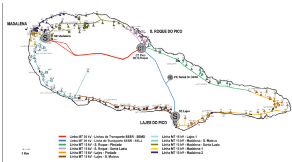
Figura 2-16 – Mapa das redes elétricas da ilha do Pico a 31/12/2023
