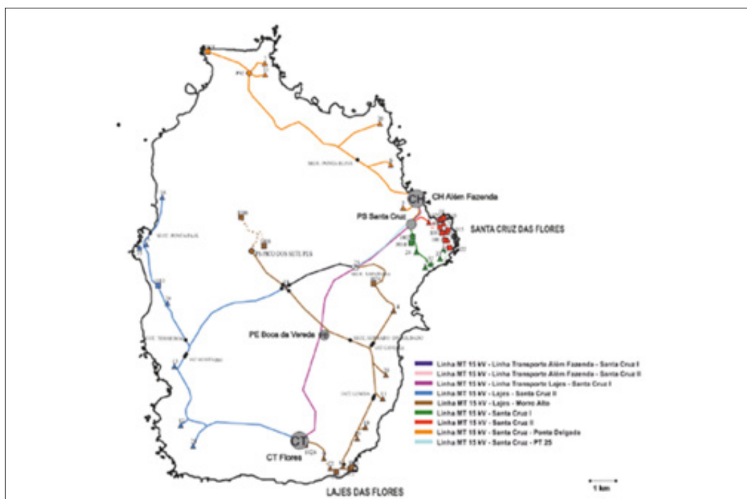
Figura 2-18 – Mapa das redes elétricas da ilha das Flores a 31/12/2023
