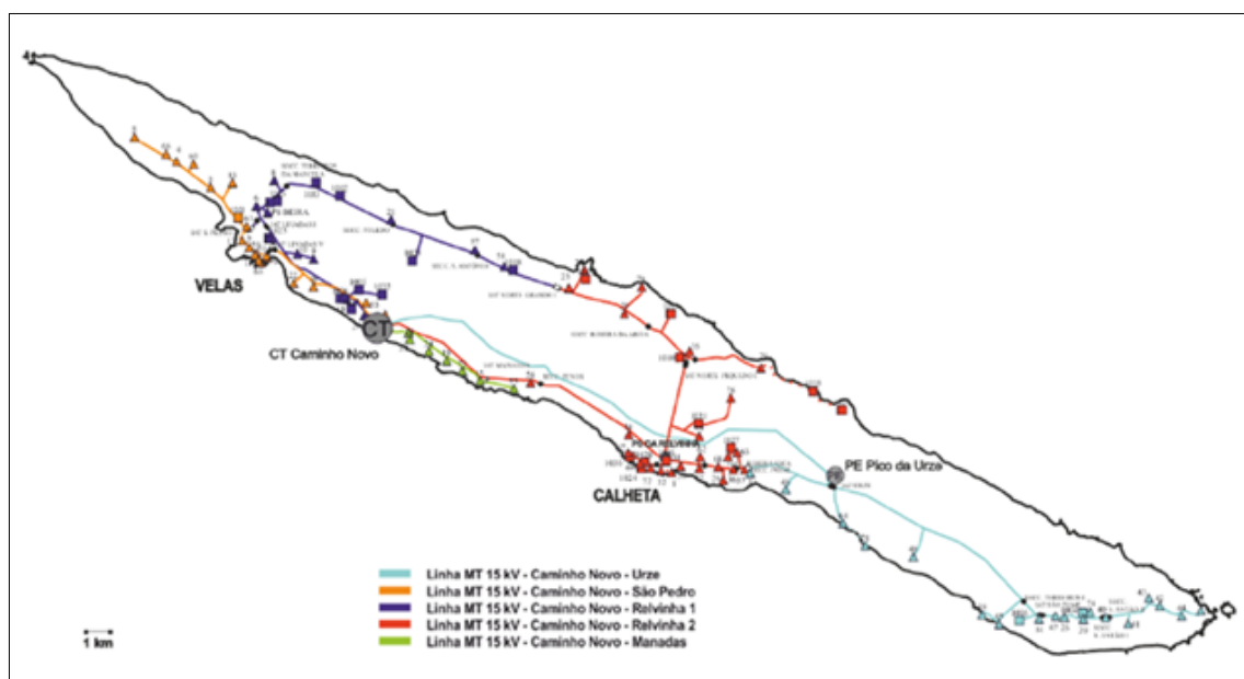
Figura 2-15 – Mapa das redes elétricas da ilha de São Jorge a 31/12/2023
