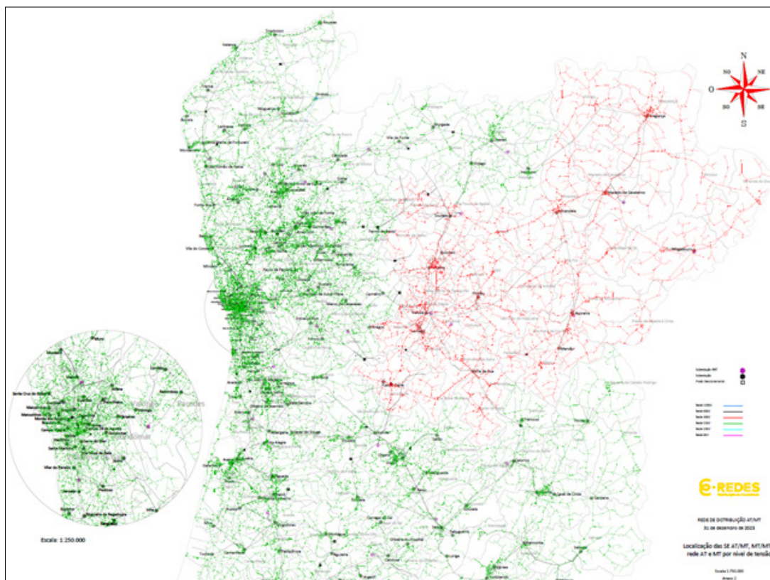
Figura 2-5 – Mapa da Rede Nacional de Distribuição a 31/12/2023 – Zona 1
