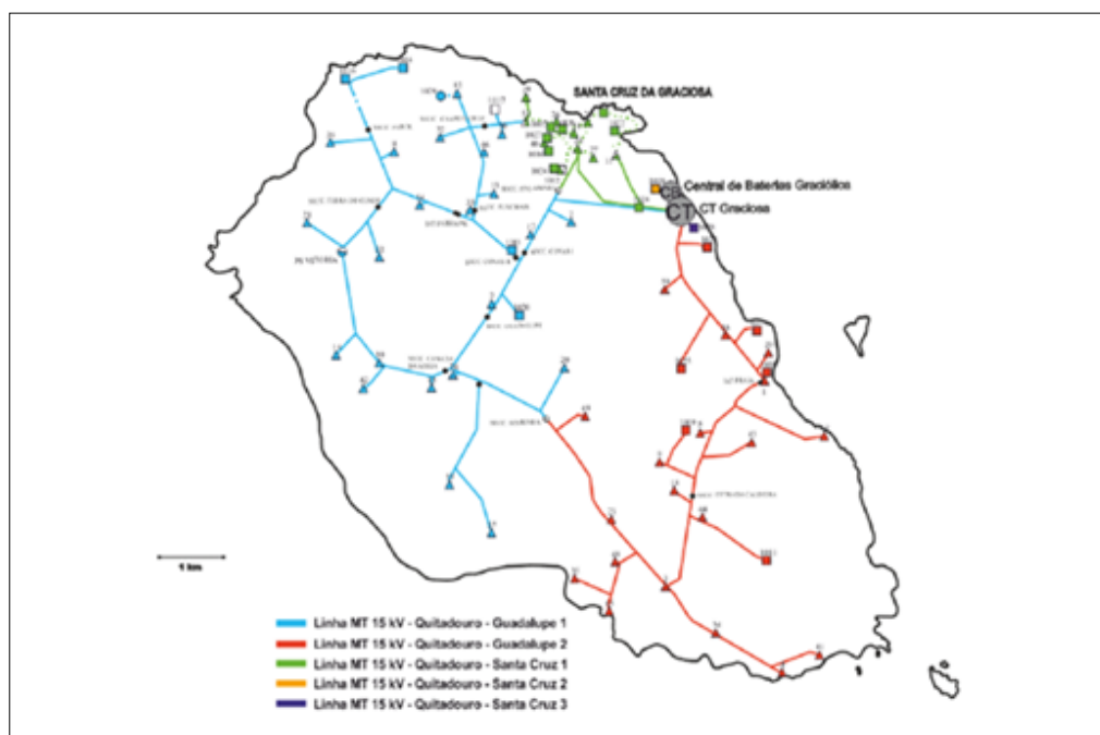
Figura 2-14 – Mapa das redes elétricas da ilha Graciosa a 31/12/2023
