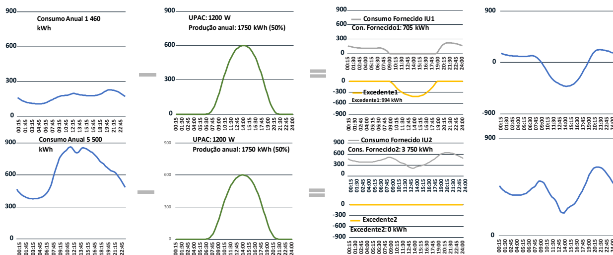
Figura 5-8 – Exemplo de apuramento dos consumos e excedentes num autoconsumo coletivo
