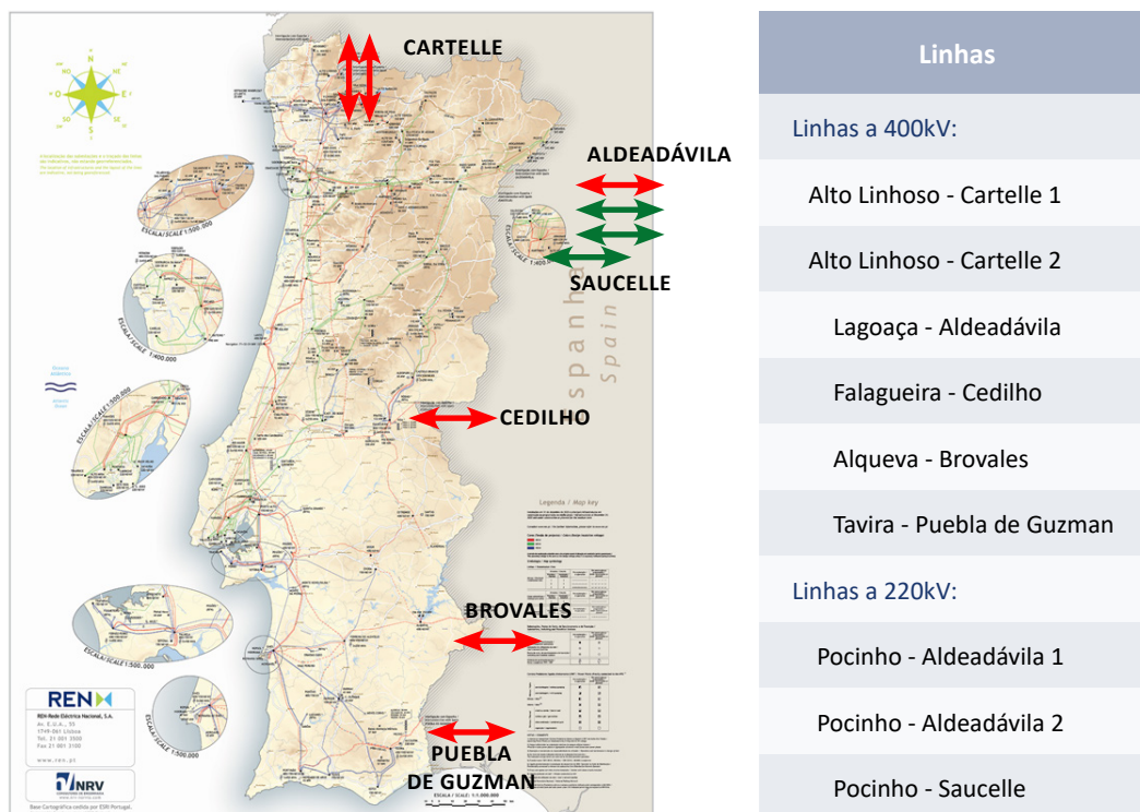
Figura 2-2 – Linhas da interligação entre Portugal e Espanha
