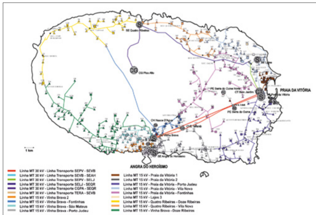
Figura 2-13 – Mapa das redes elétricas da ilha Terceira a 31/12/2023
