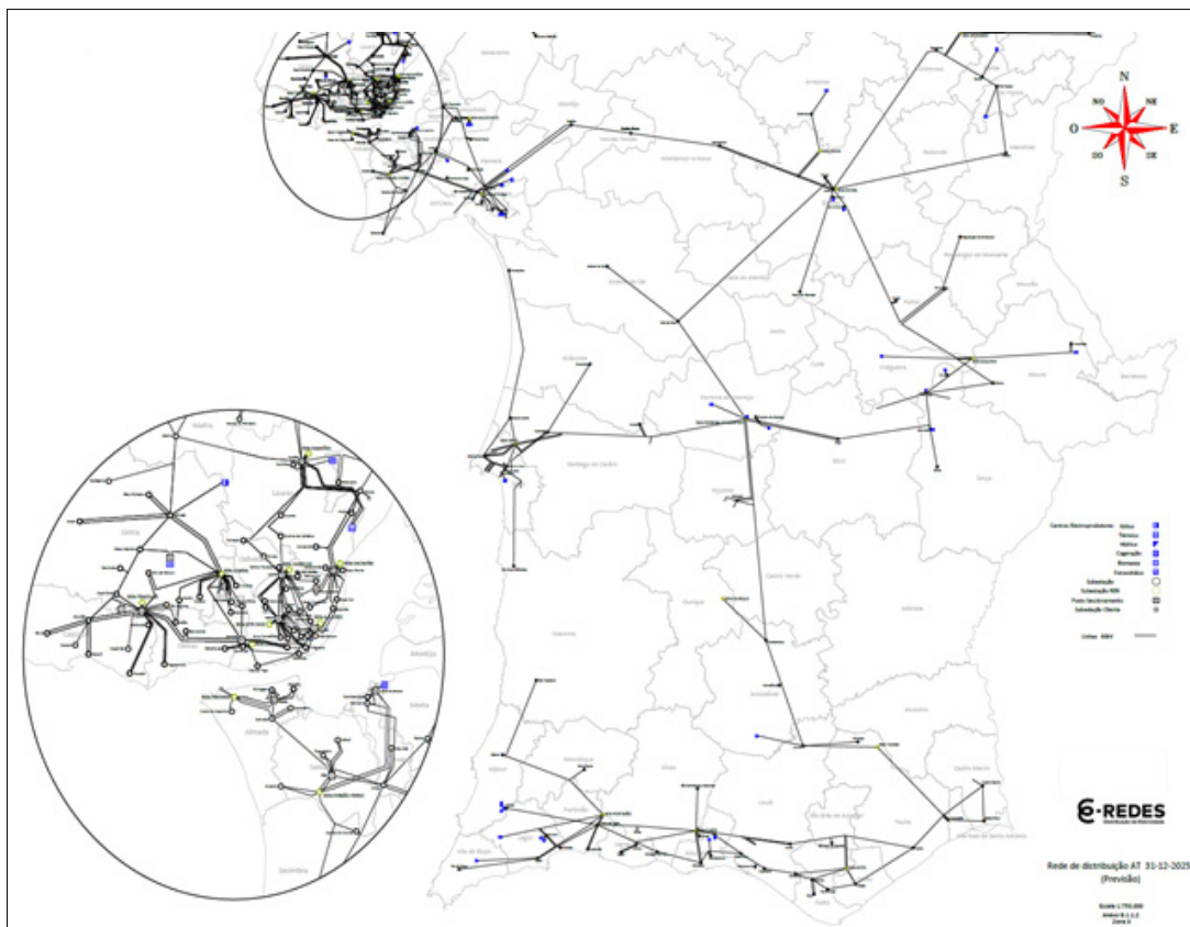
Figura 2-23 – Mapa da rede de distribuição AT e subestações AT/MT (previsão 2025) – zona 3
