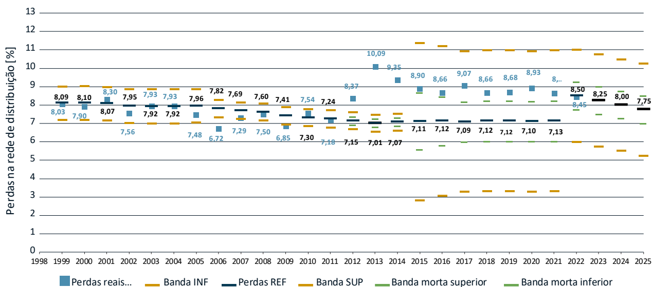
Figura 6-21 - Evolução das perdas verificadas nas redes de distribuição no referencial de entrada
