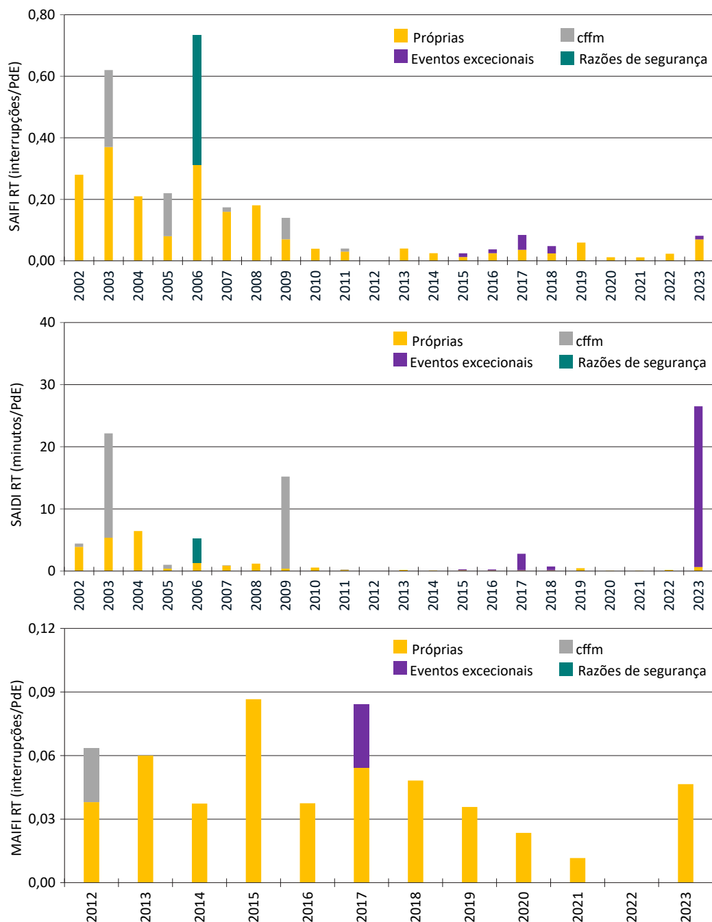
Figura 2-58 – Evolução dos principais indicadores gerais de continuidade de serviço da RNT
