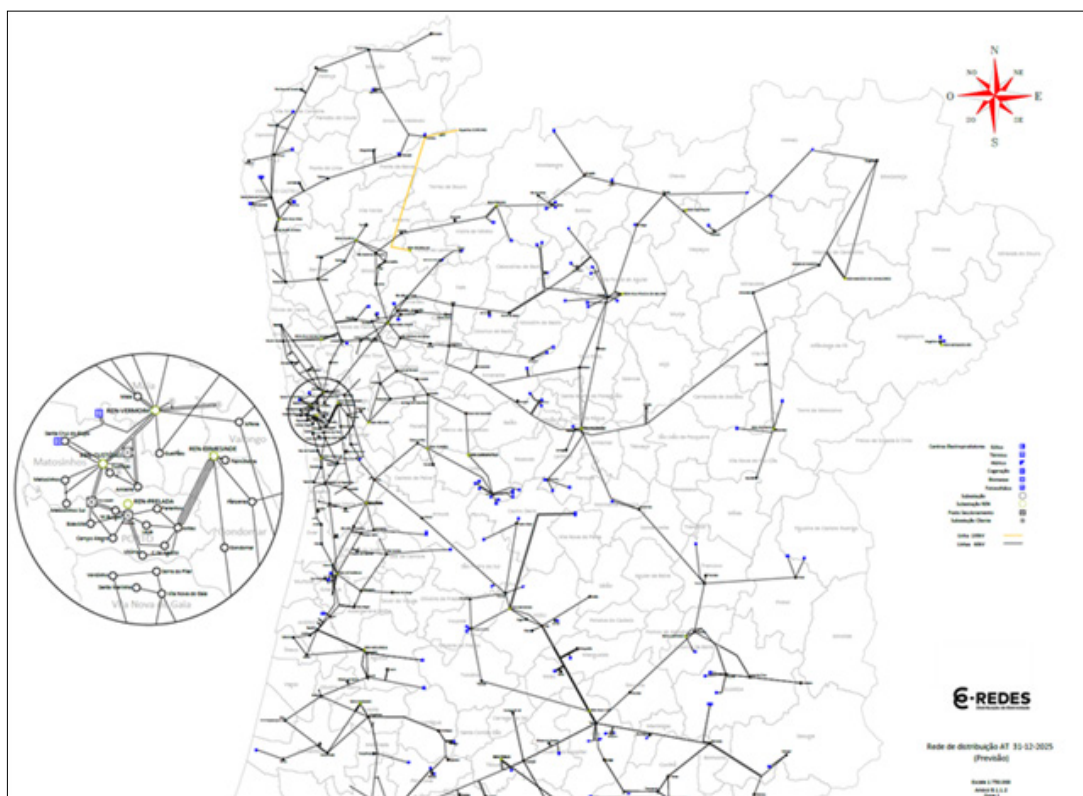
Figura 2-21 – Mapa da rede de distribuição AT e subestações AT/MT (previsão 2025) – zona 1
