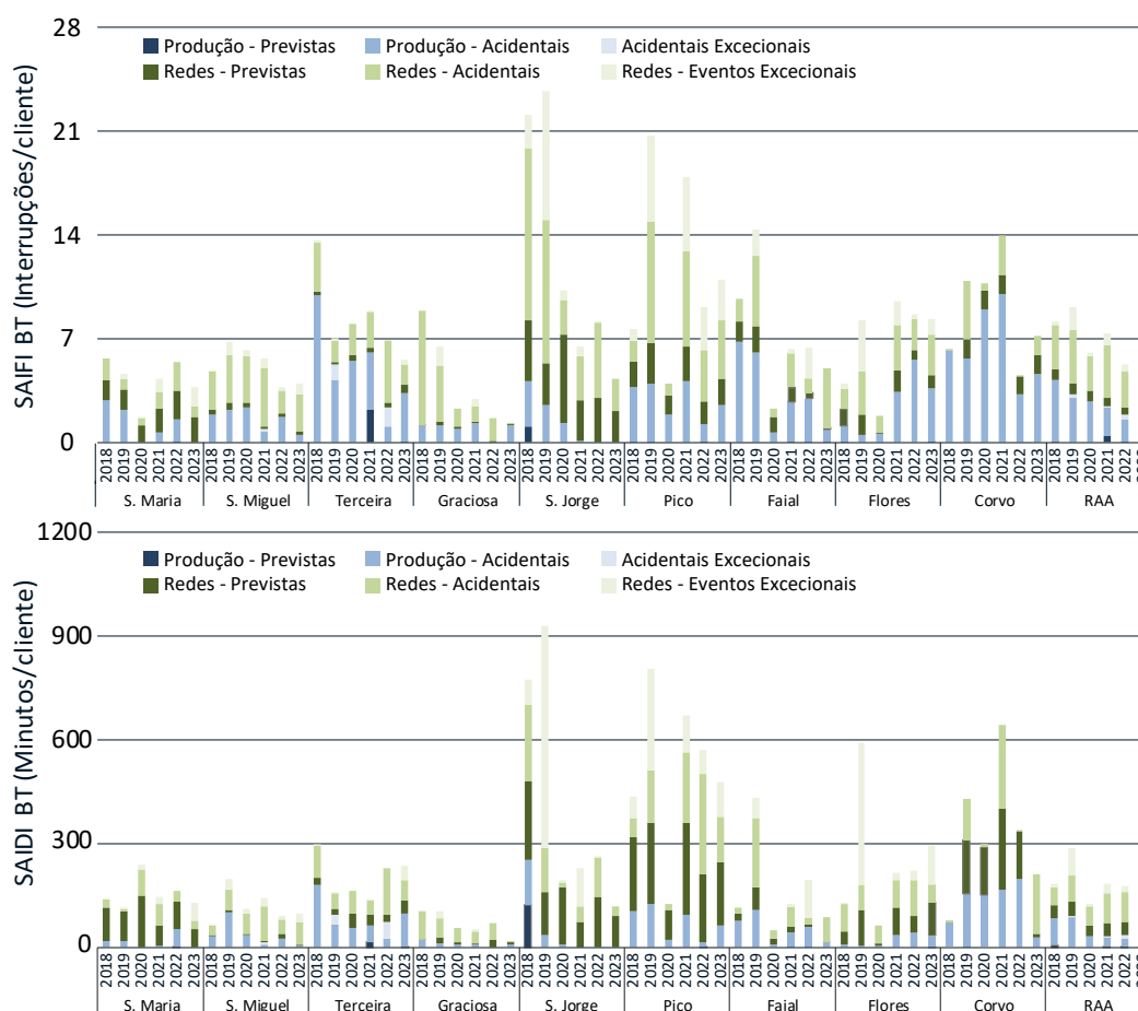
Figura 2-66 – Evolução dos principais indicadores gerais de continuidade da rede BT na RAA
