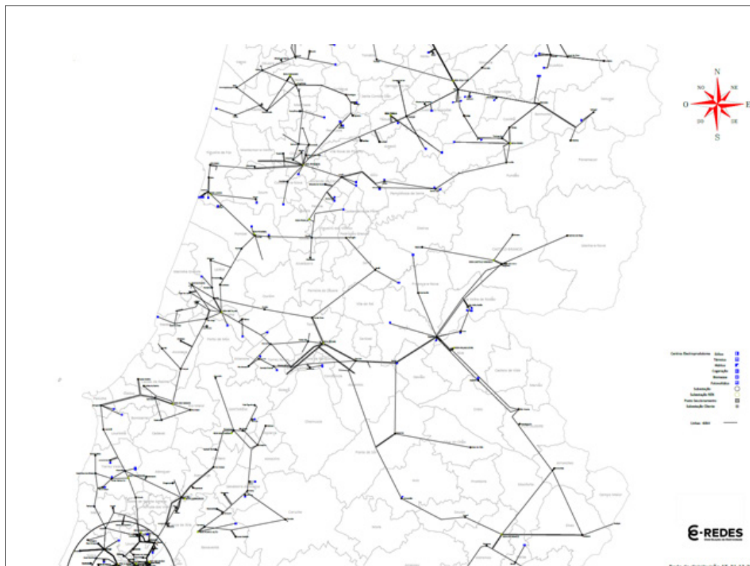
Figura 2-22 – Mapa da rede de distribuição AT e subestações AT/MT (previsão 2025) – zona 2
